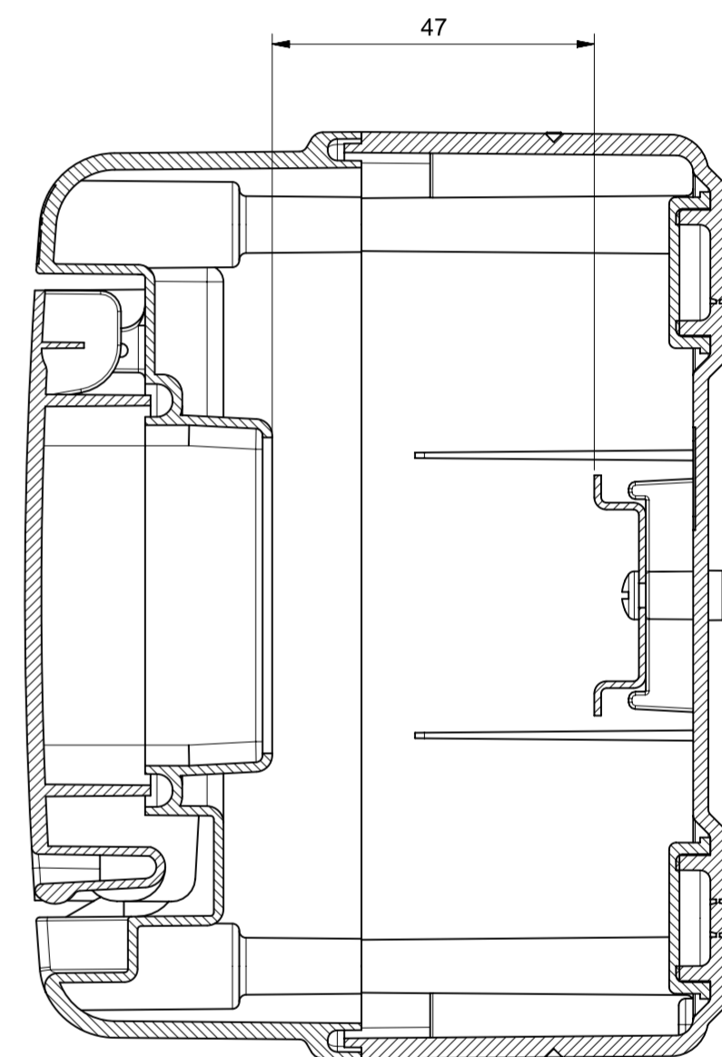
Sezione A-A
